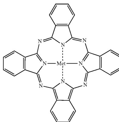
Met = Cu, Mg, AlCl, TiO 2 , SnCl 2 , etc. Met-Pc
