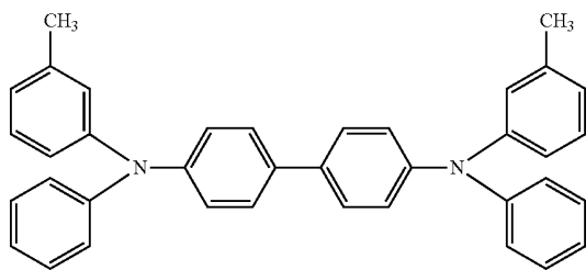
TPD
