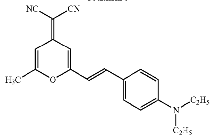
DCM-1
