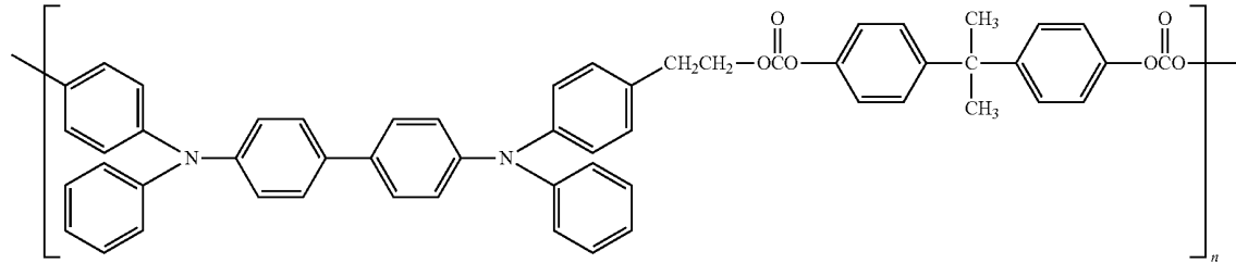
TPD-PCA
