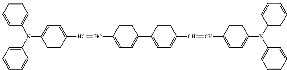
DPABVi
