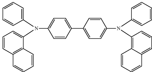
a-NPD
