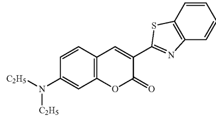
Coumarin 6
